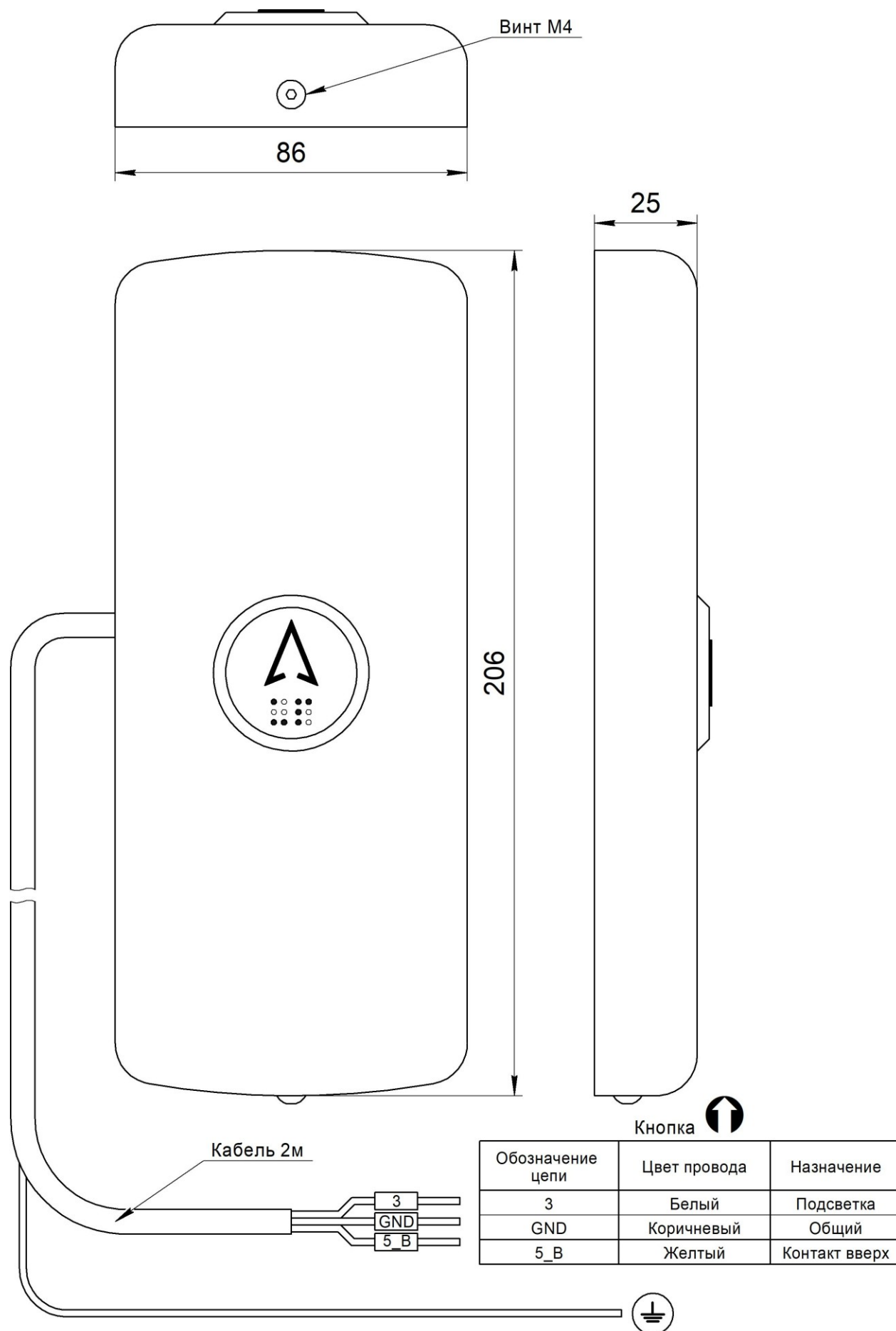
Рис.1 Внешний вид и габаритные размеры Вызывного поста ВП-1101-03
